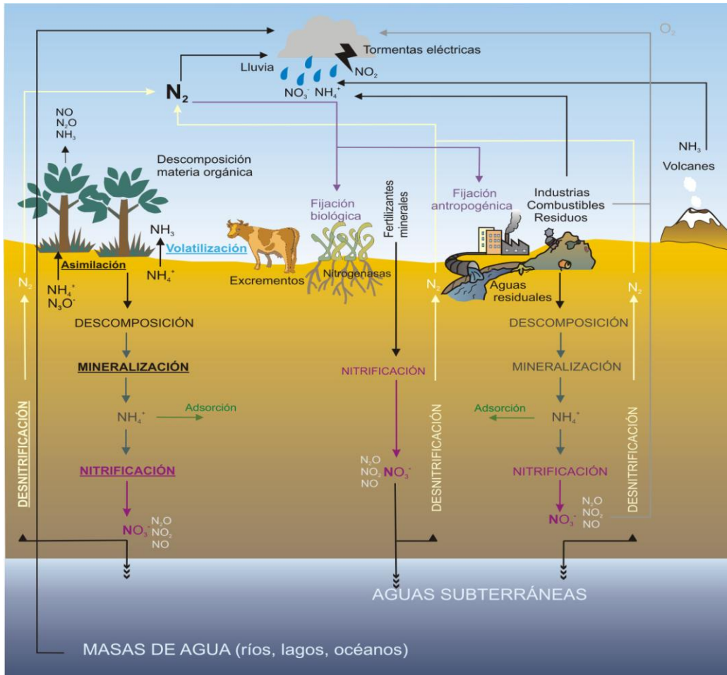
Figura 3. Fases del ciclo del Nitrógeno.
