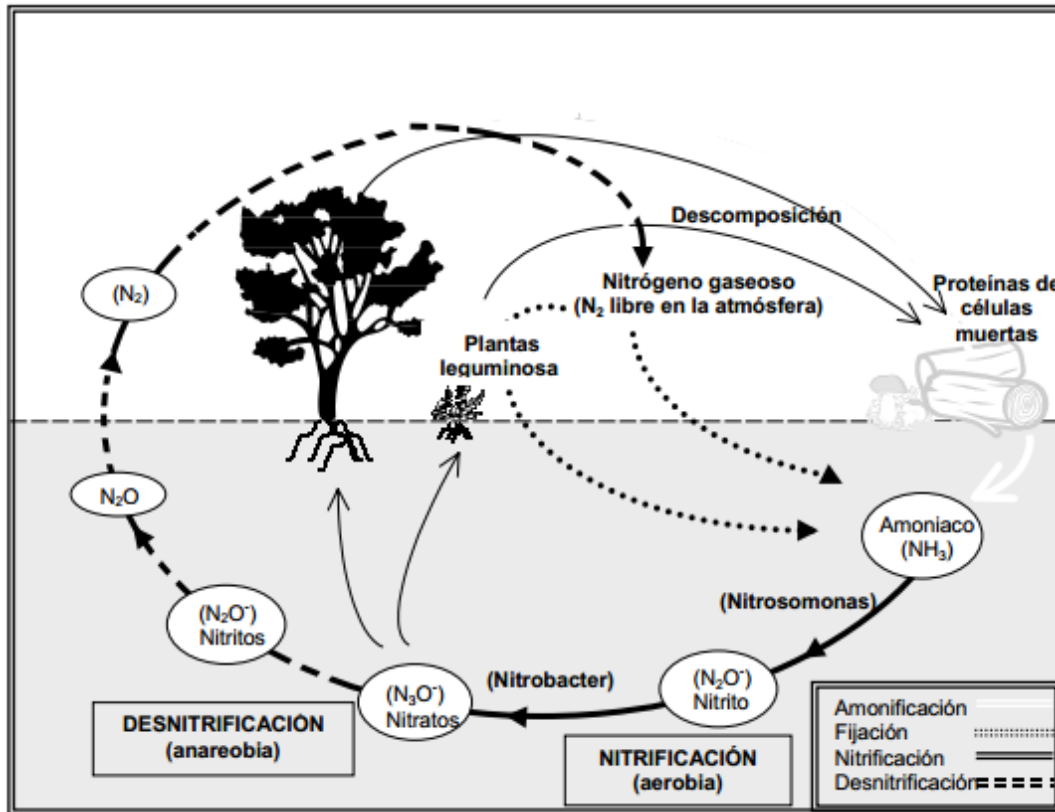
Figura 4. Ciclo de los nitratos.
